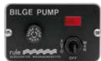
Automatischer Schalter 3 Positionen: Automatic, Manual und Off. Mit Kontrolllampe und Sicherung, 12 V. Masse: 82 x 50 mm
