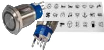
Schalter und Druckschalter mit LED 12 V, max 5 A. LED Beleuchtung anschliessbar für Schalter oder Funktion. Masse: Ø 19 mm, Länge 33 mm
