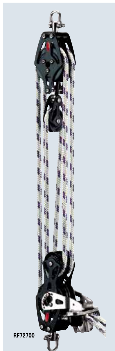
Flaschenzug Mit Übersetzung 3:1 und 6:1
