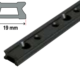
19 Schienen aus schwarz eloxiertem Aluminium, Serie 19 Für Grossschot- und Fockschlitten
