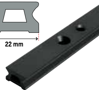
22 Schienen aus schwarz eloxiertem Aluminium, Serie 22 Für Grossschot- und Fockschlitten
