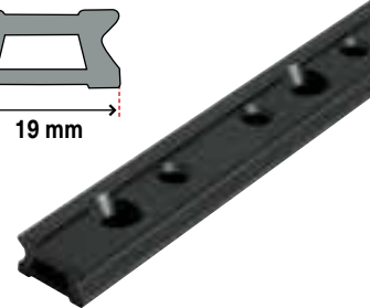
19 Schienen aus schwarz eloxiertem Aluminium, Serie 19 Für Grossschot- und Fockschlitten
