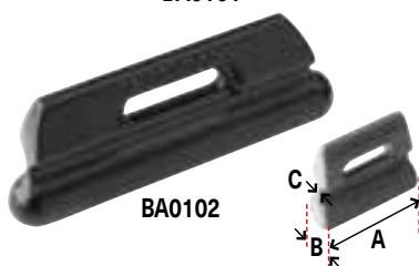
Grossbaum-Rutscher für Yachten Aus Aluminium mit Teflon®-Beschichtung
