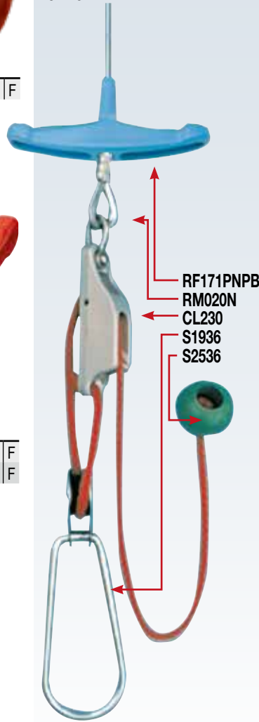
Trapezring Auf Kugellager zur Höheneinstellung. Aus rostfreiem Stahl
