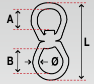
Emerillons de mouillage (utilisables en immersion permanente)
