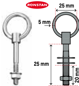
Piton à anneau mobile En acier inox Filetage: 1/4" Whitworth BSW (6 mm)
