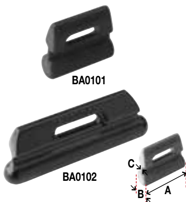
Coulisseaux de bôme pour lestés En aluminium recouvert de Teflon®
