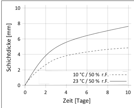
Diagramm 1: Durchhärtengeschwindigkeit Sikaflex®-521 UV
