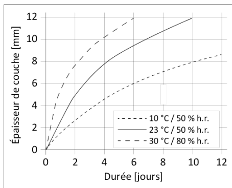
Diagramme 1: Vitesse de durcissement de Sikaflex®-252
